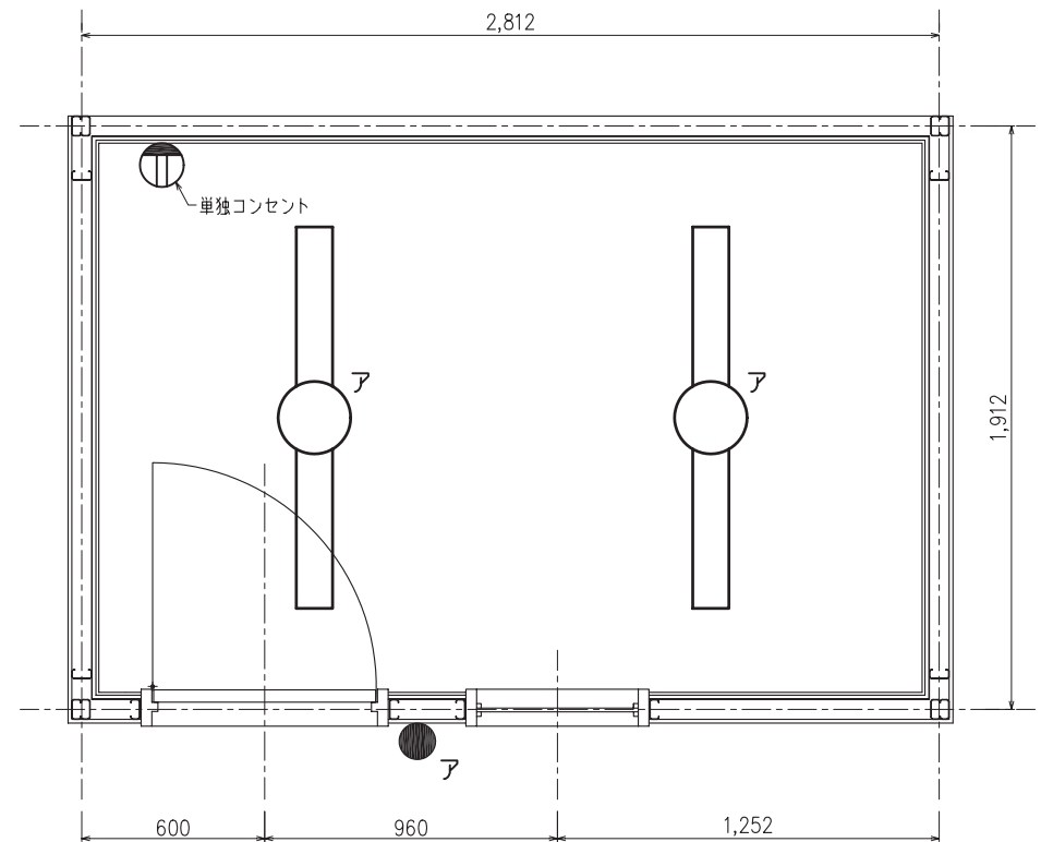
照明・コンセント配置図
